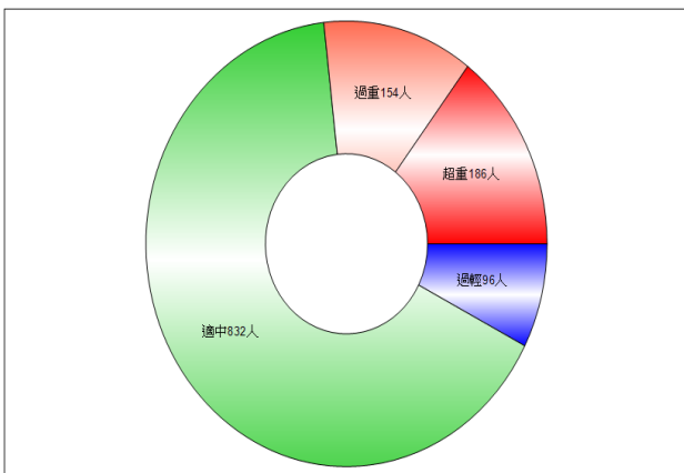
體位統計圖
